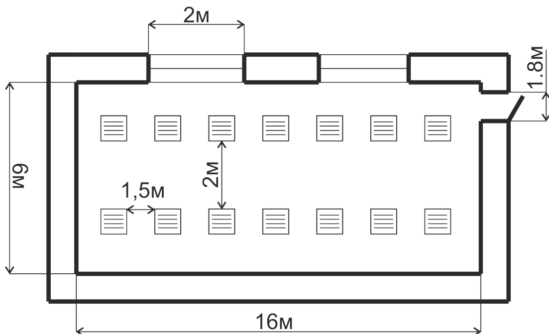
Рис. 2 Схема размещения светильников в офисе здания представлена.
